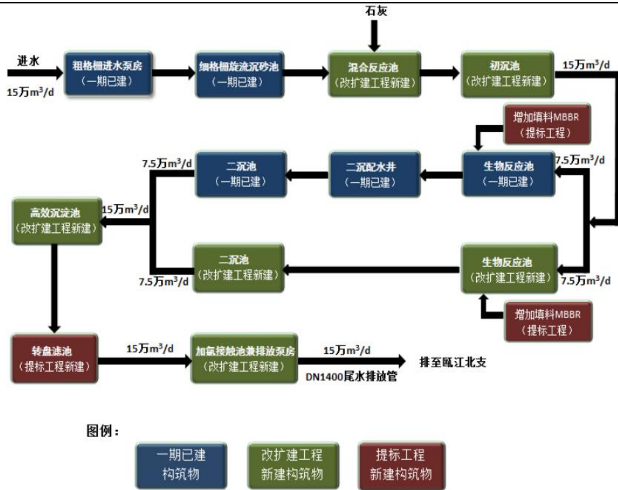
图 4-2 水处理工艺流程示意图
