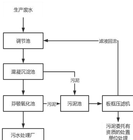
图 4-1 项目生产废水处理工艺流程示意图
