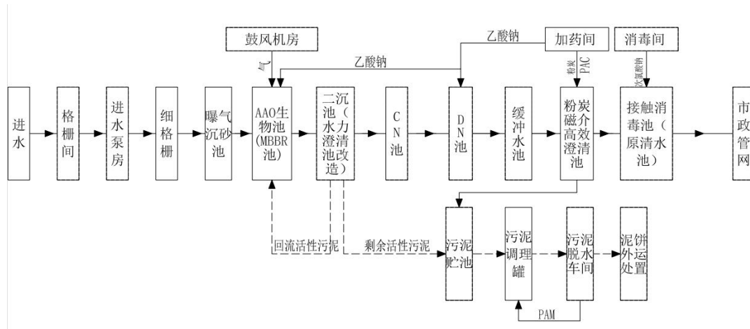
图 4-2 污水处理工艺流程示意图
